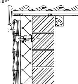
DETAIL 6A - Nieuwbouw gevelbekleding topgevel onder de kantpannen aansluiten met ventilatie
