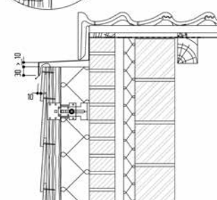
DETAIL 6B - Renovatie dichting tussen gevelbekleding topgevel en kantpannen d.m.v. geplooiden metalen driuplijst.
