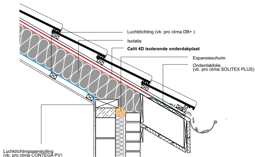
Doorsnede boven: betimmering op keperplanken. Foto onder: variante.
