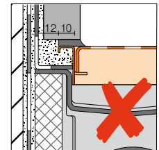
Montage incorrect (Fig. Cadre standard)
