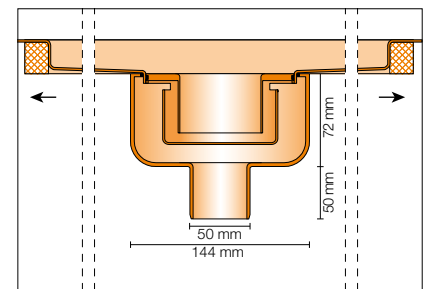
Coupe longitudinale – Montage le long d'un mur et montage au centre de la douche
