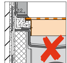
Montage incorrect (Fig. Cadre discret)
