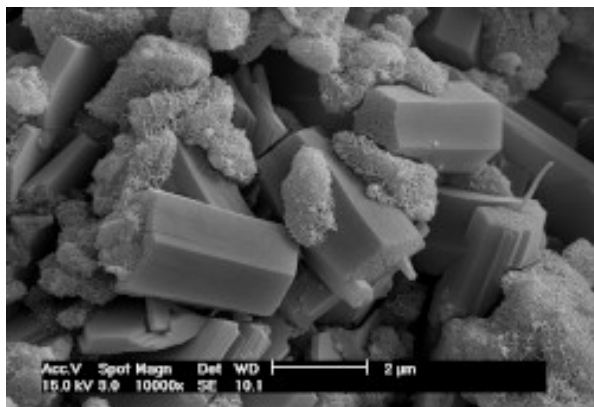
Hydratation d' Ultracolor Plus , liant spécial à base de ciment. Notez l'absence de cristaux lamellaires de ciment Portland (hydroxyde de calcium), qui est la cause de l'efflorescence blanchâtre
